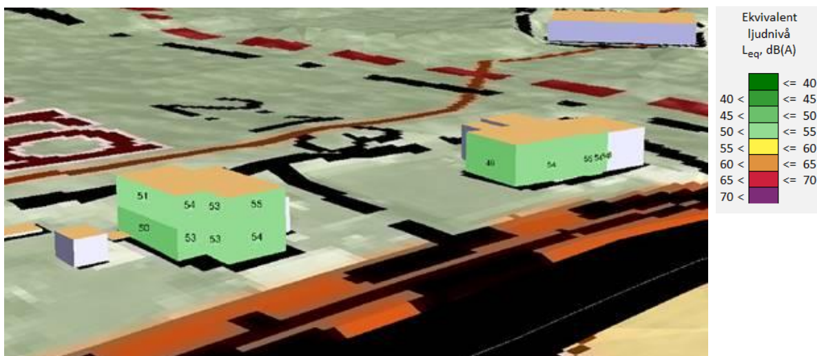
Figur 10: Ekvivalent ljudnivå vid fasad, Flyttad väg 15m. (Notera att skalan anpassats så gult avser över 55dB(A))
